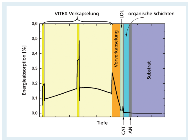
Absorbierte Elektronenenergie in einem typischen OLED-Schichtstapel
